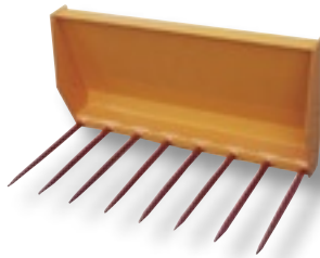
Dunggabel Breite: 1,25m - 2,35m Zinkenlänge: 800mm/ 1000mm
