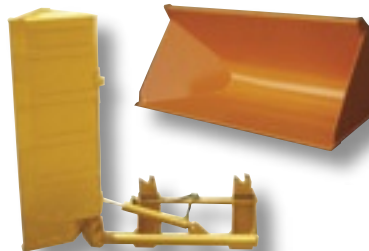
Seitenkippschaufel rechts- oder linkskippend Breite: 1,60m - 2,30m Inhalt: 0,48m 3 - 0,83m 3
