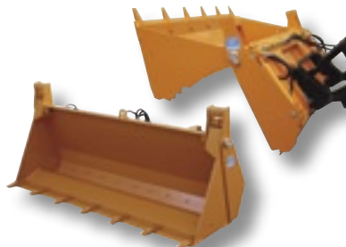
Greifschaukel „4in1“ verstärkte Ausführung Breite: 1,60m - 2,30m Inhalt: 0,57m 3 - 0,80m 3
