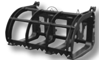
Poltergabel - extra verstärkt - 4 bzw. 5 Zinken, langer Greifer Breite: 1,60m / 1,80m / 2,00m Zinkenlänge: 1000mm/ 1200mm
