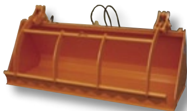
Schwergutschaufel mit Greifer Breite: 1,60m - 2,30m Inhalt: 0,8m 3 - 1,2m 3 Greifer mit Zackenleiste oder Zinken
