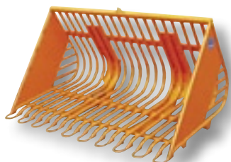
Rübenkorb, absolut fruchtschonend Rohrabstand: ca. 65mm Breite: 1,60m - 2,50m Inhalt: 1,00m 3 - 1,60m 3
