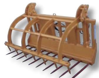
Vielzweckgabel Breite: 1,20m - 2,35m Zinkenlänge: 800mm / 1100mm
