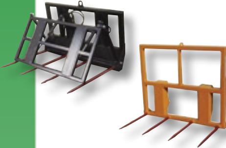
Großballengabel Rahmenausführung, Großballengabel mit Abschieber Breite: 1,80m - 2,00m Zinkenlänge: 1250mm / 1400mm a.W. Rahmenerhöhung: bis 2,50m
