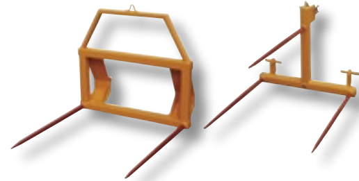
Großballengabel , für Frontlader oder Heckanbau Zinken: 2 oder 3 Zinkenlänge: 1100mm/ 1400mm
