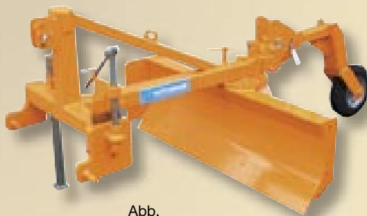
Abb. u.a. Zusatzausrüstung - Neigungsverstellung 15° - Tastrad-Mitte, höhenverstellbar
